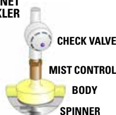
VIBRONET SPRINKLER
