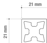
Upright 7711
