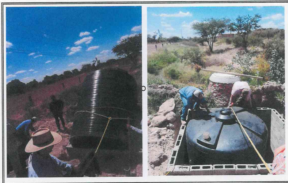
CONSTRUCCION DE FOSA SEPTICA CON BIODIGESTOR DE CAPACIDAD DE 7,500 LITROS PARA BENEFICIAR A 18 VIVIENDAS EN LA COMUNIDAD DE AGUAGORDA, VILLA GARCIA, ZACATECAS
