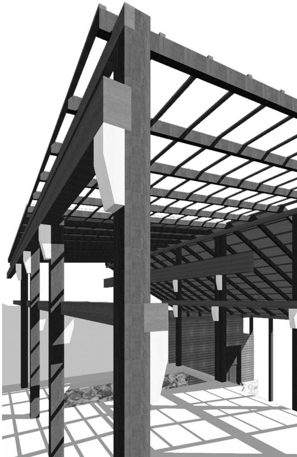
Figura 11. Detalle de la casa de máquinas en la hacienda de San Antonio Tehuizt. Fuente: Roberto Reyes.
