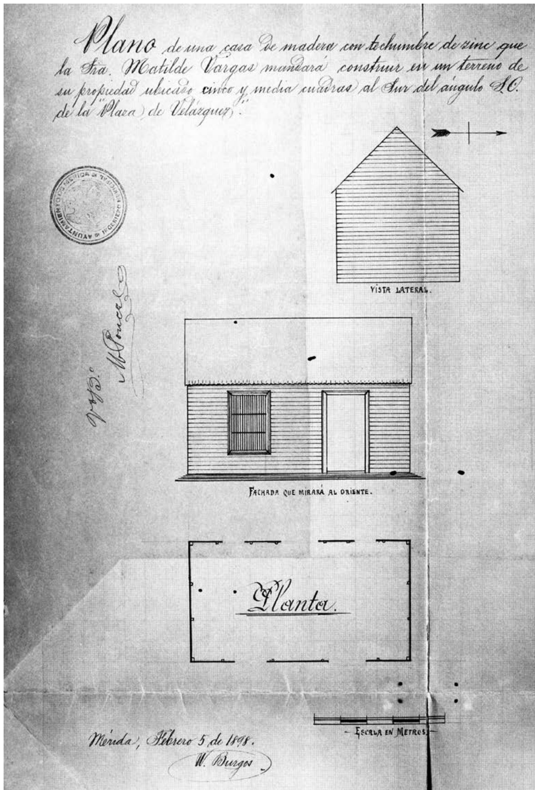
Figura 7. Plano de una casa de madera para la señora Matilde Vargas, a construirse en el suburbio de Santiago, 1898. Fuente: Biblioteca Virtual de Yucatán.
