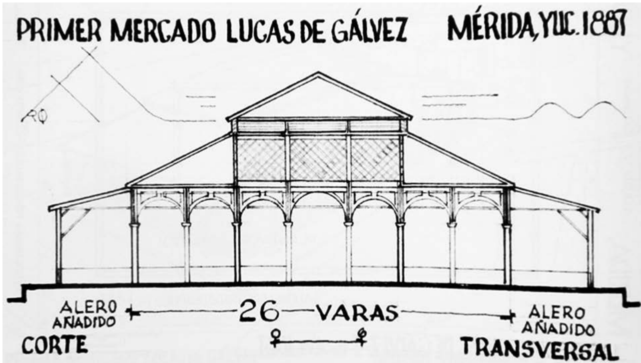
Figura 5. Corte del primer mercado Lucas de Gálvez, donde se aprecian los arcos de madera, las celosías y los tapancos, así como las ventilas superiores. Fuente: Arcel Espadas Medina, El modernista bazar-mercado de Mérida. De la modernización yucatanense-porfirista, 1880 , Mérida, UADY/INAH, 2010.
