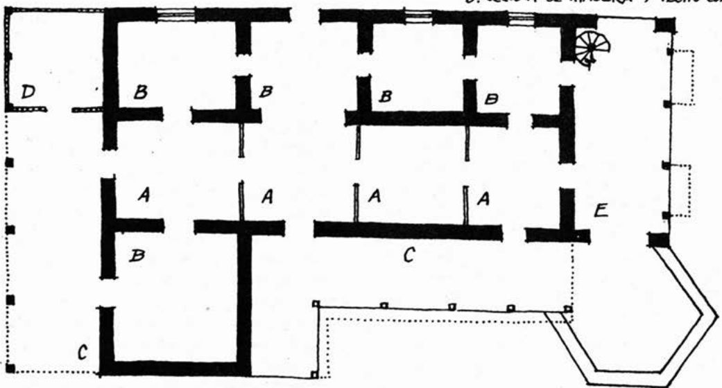
FIGURA 7. Planta y apunte en perspectiva de una casa del Tipo 5 en Itzimná, ciudad de Mérida; 1900 ca.
