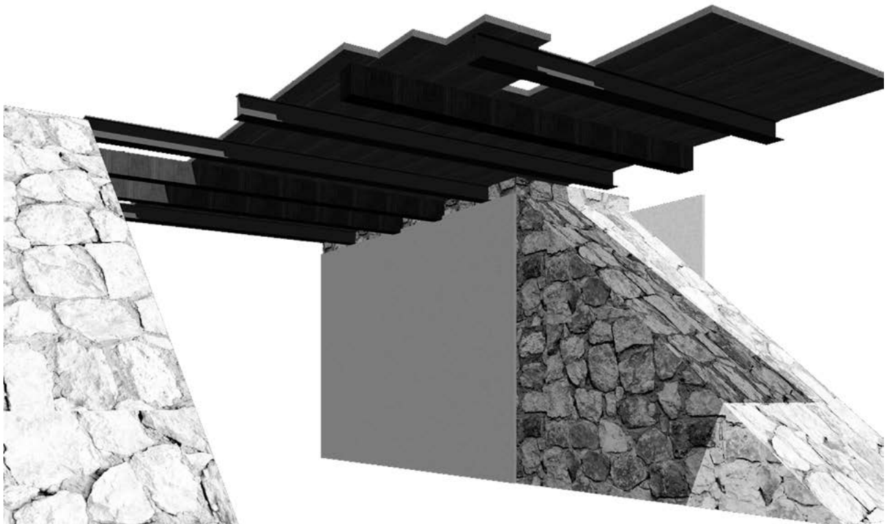
Figura 14. Detalle de bagacera (entresuelo) en la casa de máquinas de la hacienda de Yaxché de Peón. Fuente: Roberto Reyes.
