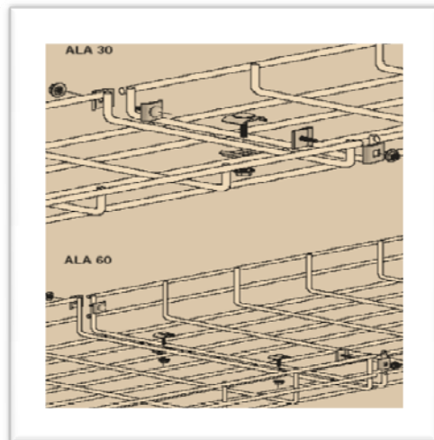
UNION DE TRAMO (SOPORTE LIGERO)
