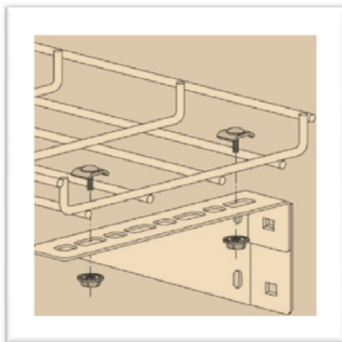
UNION DE TRAMO DE BANDEJA PORTACABLES VIAFIL A SOPORTES NO INSTA-FIX.
