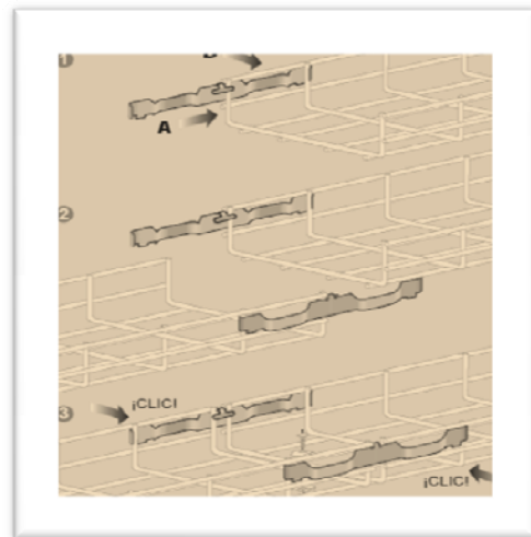
UNION DE TRAMO RECTO (SOPORTE REFORZADO)
