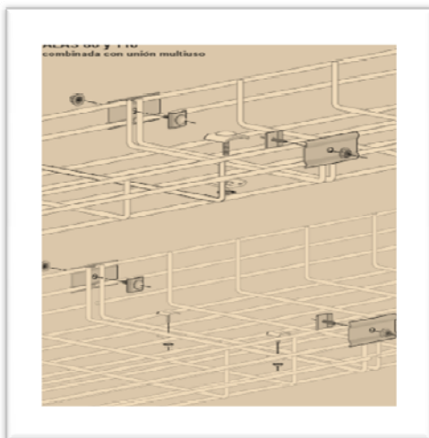
UNION DE TRAMO RECTO (SOPORTE MEDIO)
