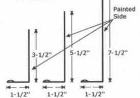
L-Trim
