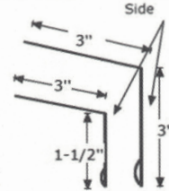
Drip Edge
