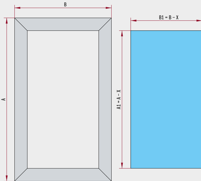
Doors with 45-degree junction - Portes avec jonction à 45 degrés Puertas con uniones de 45 grados
