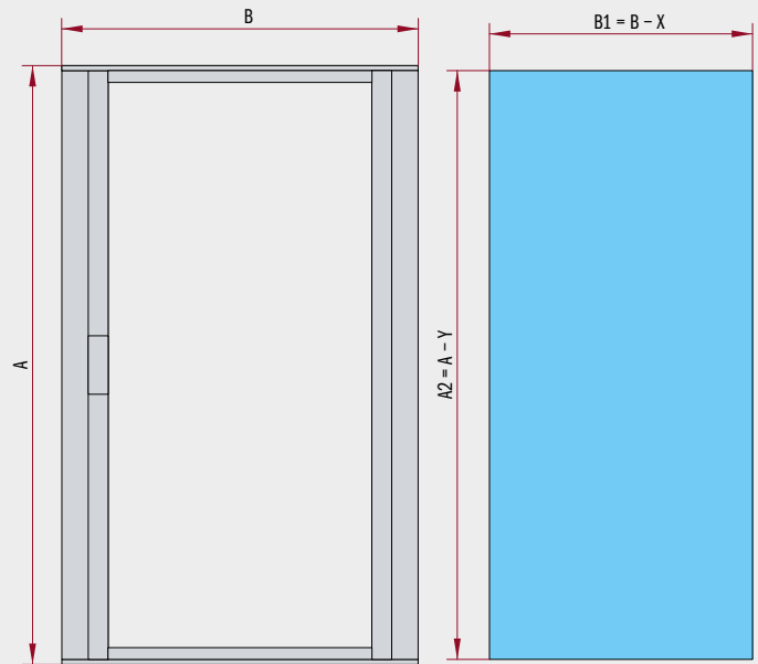
Doors with 90-degree junction - Portes avec jonction à 90 degrés Puertas con uniones de 90 grados
