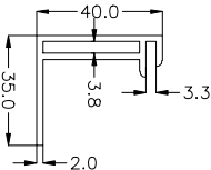
PERFIL MARCO DE MODULO SOLAR ESCALA: 1/4
