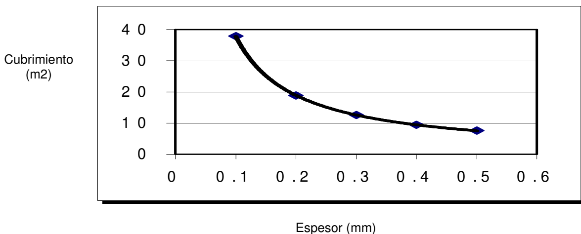
Rendimiento teórico por galón en capa líquida, superficie lisa no absorbente
