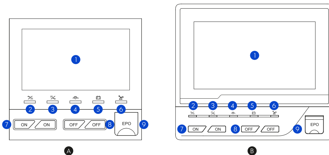
Figura 2-4 Panel de operación UPS-IND 1300 HF (A) 10~120 kVA y (B) 160~200 kVA
