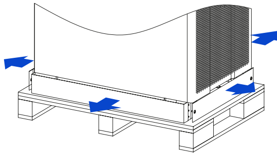
Figura 3-8 Retire las cubiertas inferiores
