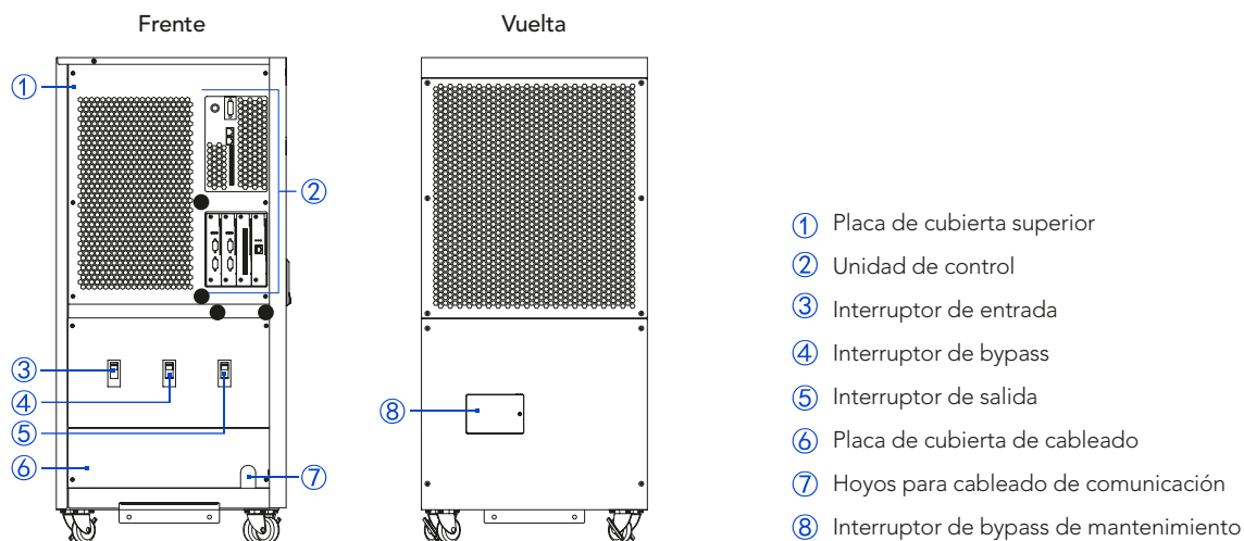
Figura 2-6 Diagrama del diseño de estructura del UPS-IND 1300 HF (50~60 kVA)
