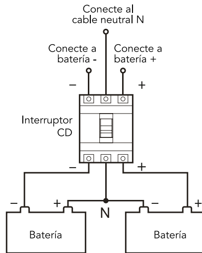
Figura 3-24 Diagrama de cableado de la batería
