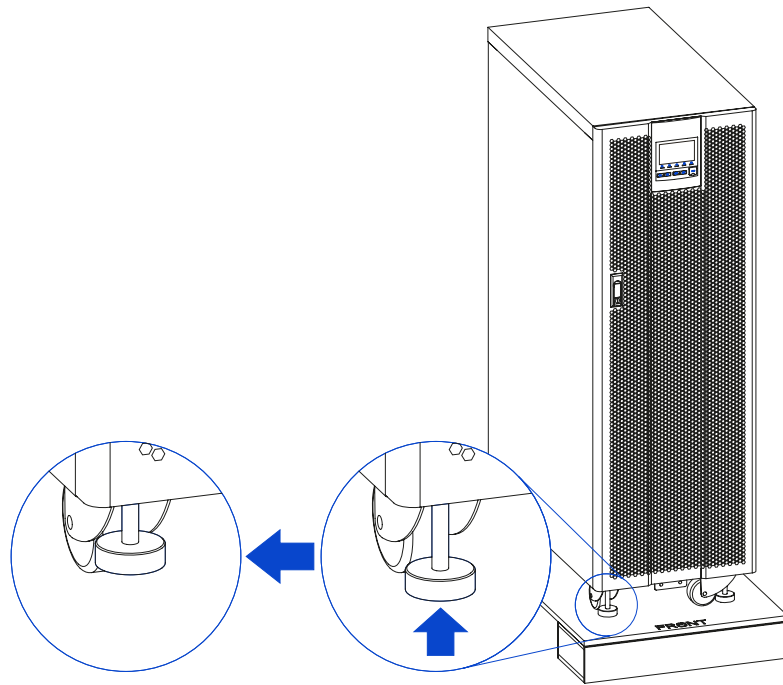
Figura 3-6 Ajuste los pies de apoyo
