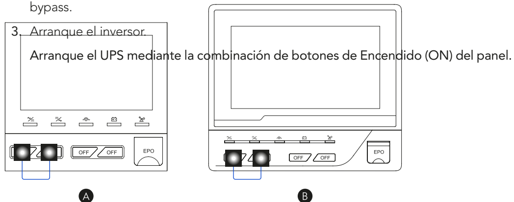
Figura 5-2 Combinación de botones ON UPS-IND 1300 HF (A) 10~120 kVA y (B) 160~200 kVA
