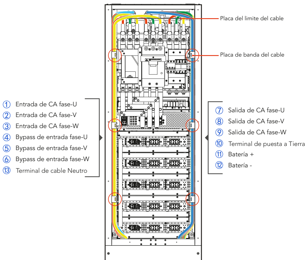
Figura 3-27 Diagrama de cableado descendente
