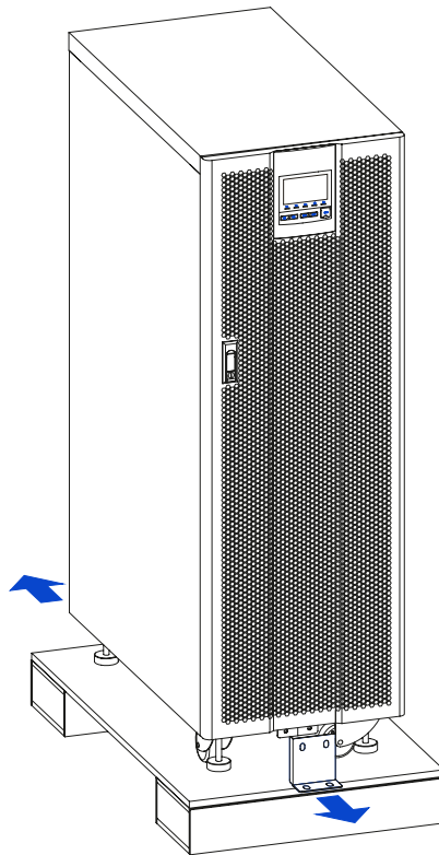
Figura 3-5 Retire las placas de soporte inferiores
