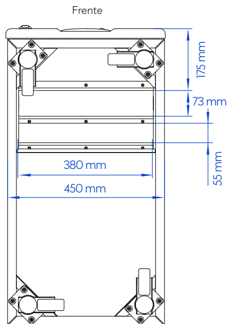
Figura 3-20 Diagrama de agujeros de cableado inferior de UPS-IND 1300 HF (80~120 kVA)
