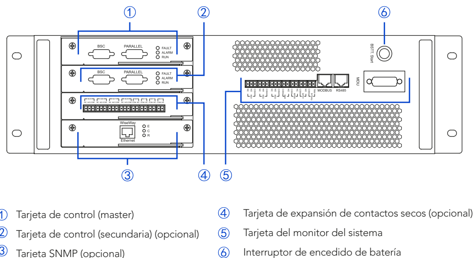
Figura 2-9 Unidad de control del UPS-IND 1300 HF (10~60 kVA)
