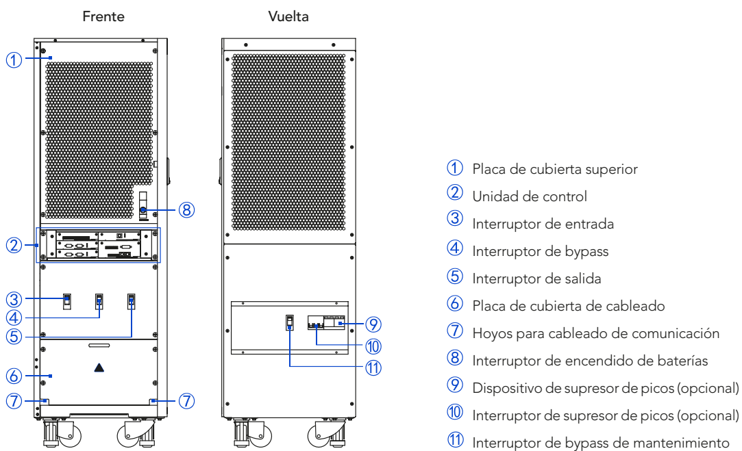
Figura 2-7 Diagrama del diseño de estructura del UPS-IND 1300 HF (80~120 kVA)
