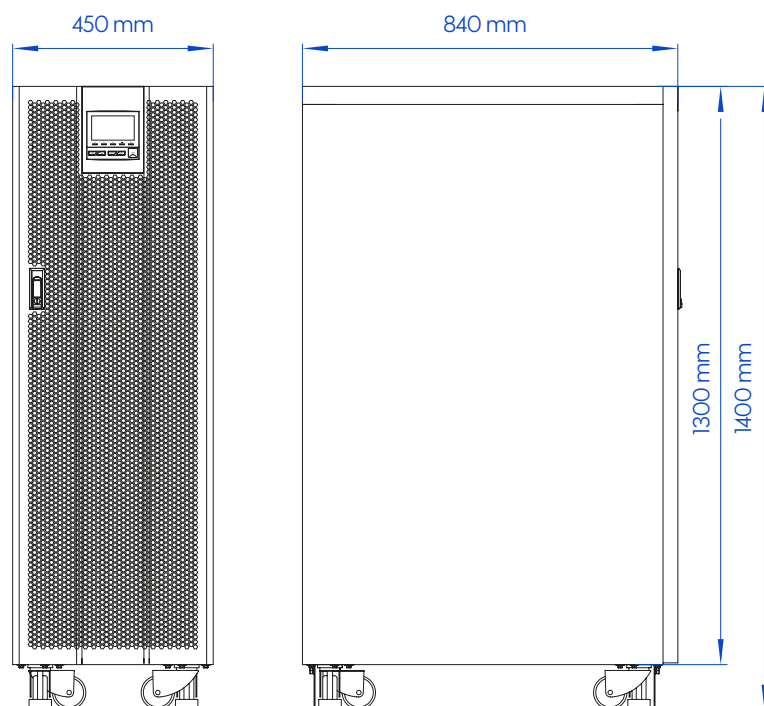
Figura 3-12 Tamaño de UPS-IND 1380 HF, UPS-IND 13100 HF, UPS-IND 13120 HF
