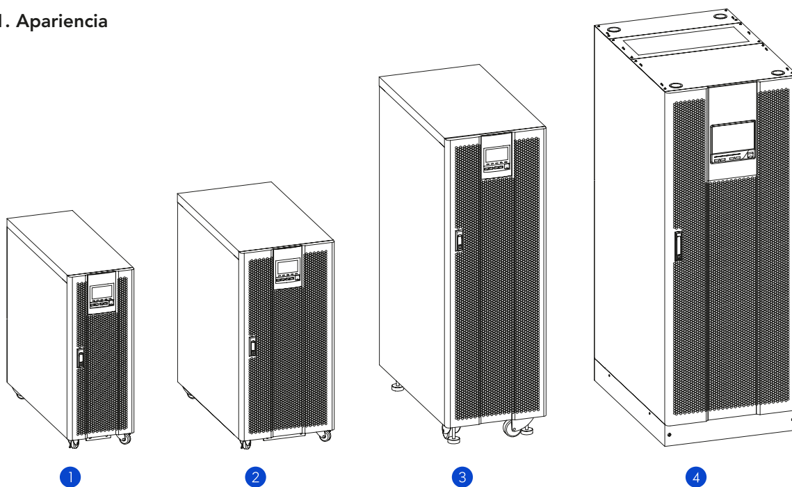
Figura 2-3 Apariencia del los diferentes modelos del UPS-IND 1300 HF (10~200 kVA)
