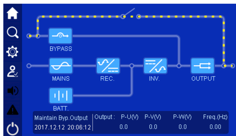
Figura 4-6 Salida de bypass de mantenimiento
