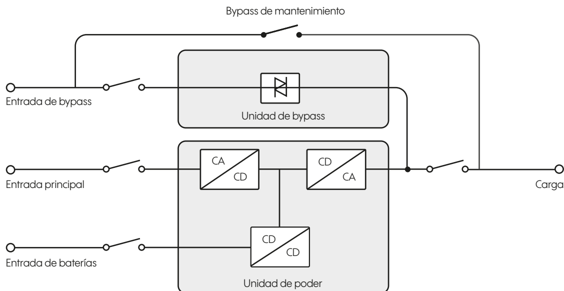
Figura 2-2 Diagrama del principio de funcionamiento
