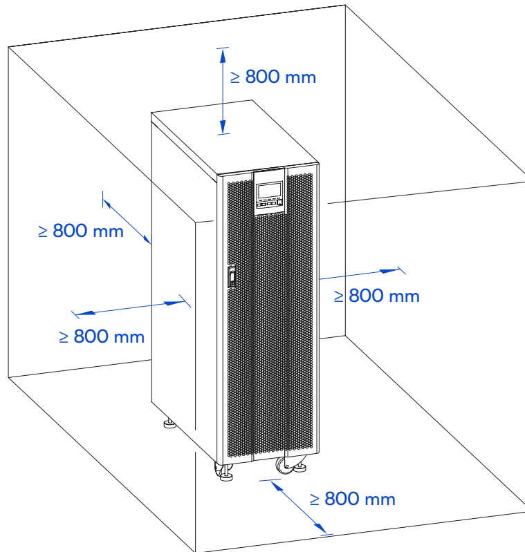
Figura 3-3 Espacio mínimo de instalación
