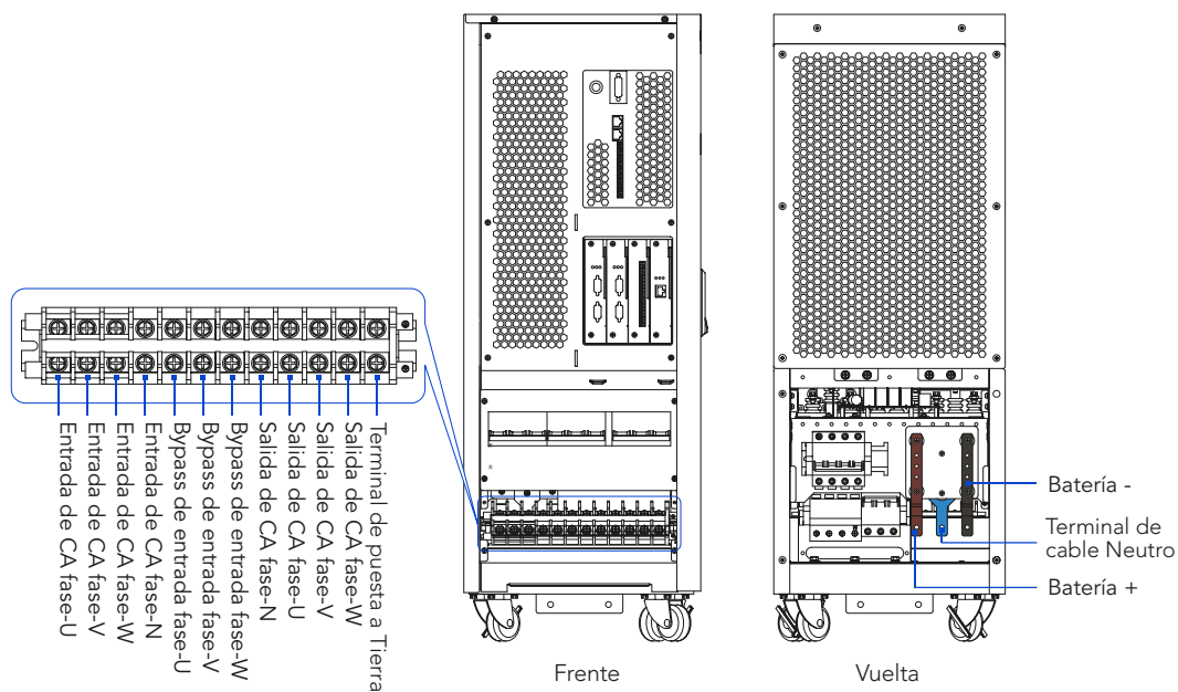
Figura 3-21 Diagrama de terminales de cableado de UPS-IND 1300 HF (10~40 kVA)
