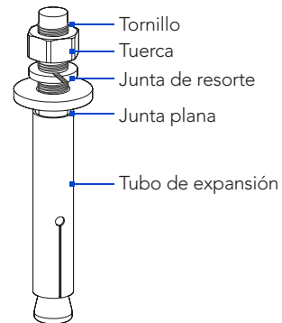
Figura 3-16 Estructura e instalación del perno de expansión
