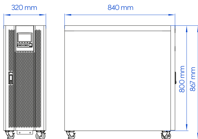
Figura 3-10 Tamaño de UPS-IND 1310 HF, UPS-IND 1320 HF, UPS-IND 1330 HF, UPS-IND 1340 HF
