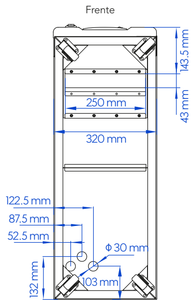
Figura 3-18 Diagrama de agujeros de cableado inferior de UPS-IND 1300 HF (10~40 kVA)
