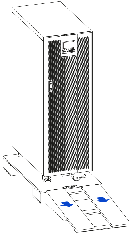
Figura 3-7 Coloque la placa deslizante.
