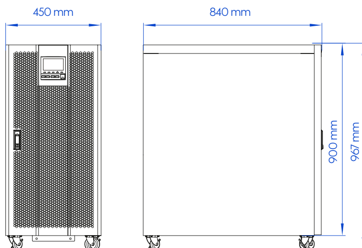
Figura 3-11 Tamaño de UPS-IND 1350 HF, UPS-IND 1360 HF
