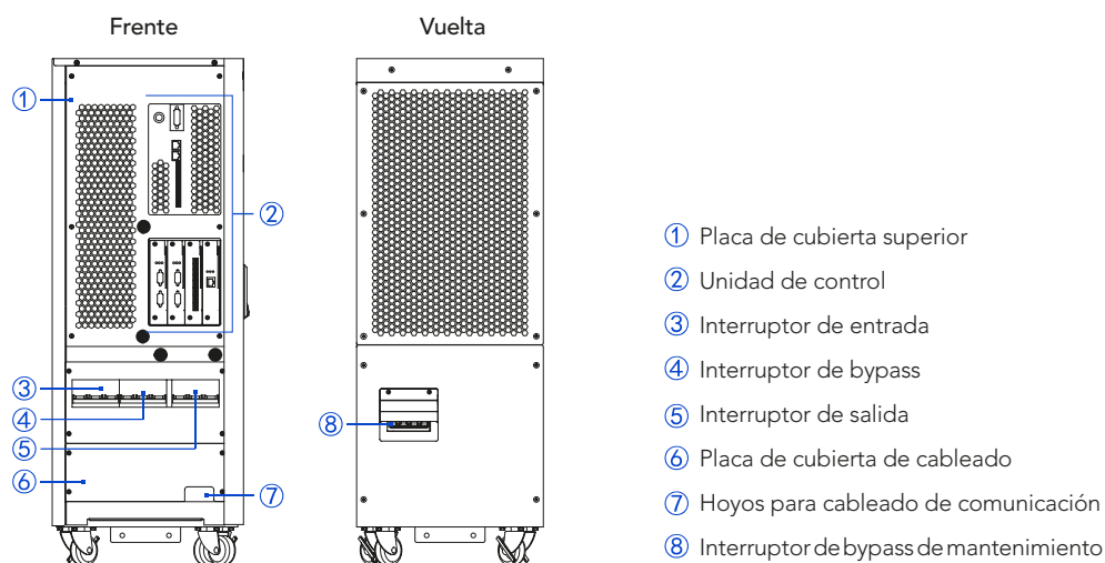
Figura 2-5 Diagrama del diseño de estructura del UPS-IND 1300 HF (10~40 kVA)
