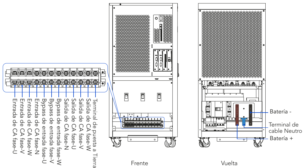
Figura 3-22 Diagrama de agujeros de cableado inferior de UPS-IND 1300 HF (50~60 kVA)
