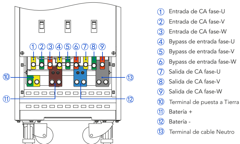
Figura 3-23 Diagrama de agujeros de cableado inferior de UPS-IND 1300 HF (80~120 kVA)
