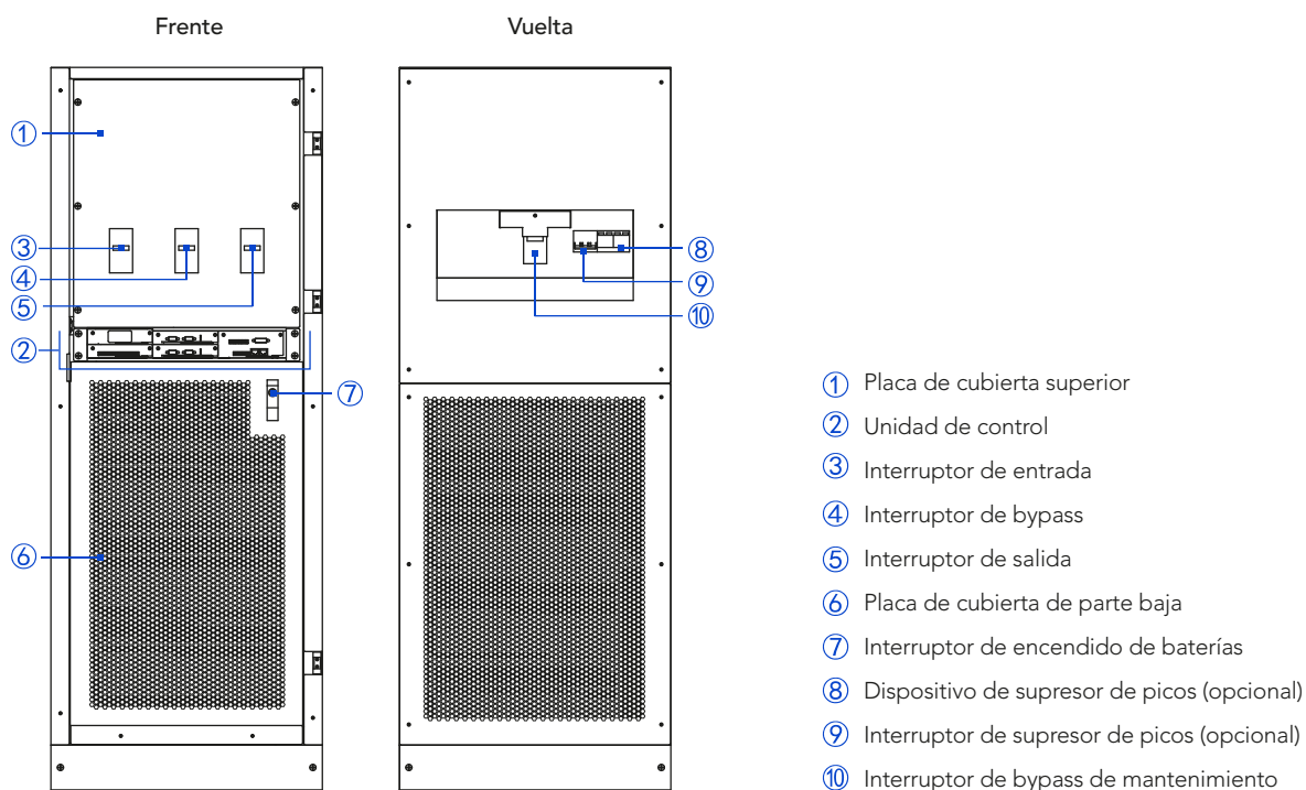
Figura 2-8 Diagrama del diseño de estructura del UPS-IND 1300 HF (160~200 kVA)
