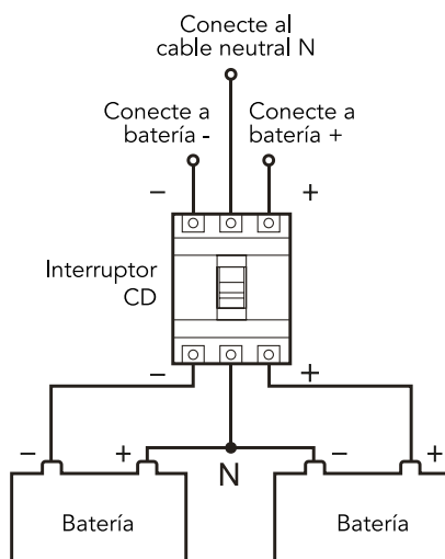
Figura 3-28 Diagrama de cableado de la batería
