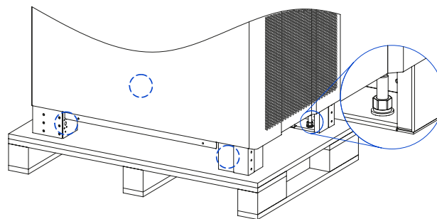
Figura 3-9 Posición de los pernos
