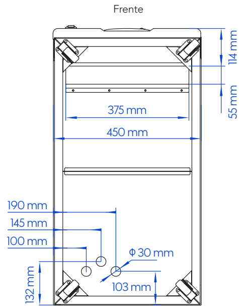
Figura 3-19 Diagrama de agujeros de cableado inferior de UPS-IND 1300 HF (50~60 kVA)
