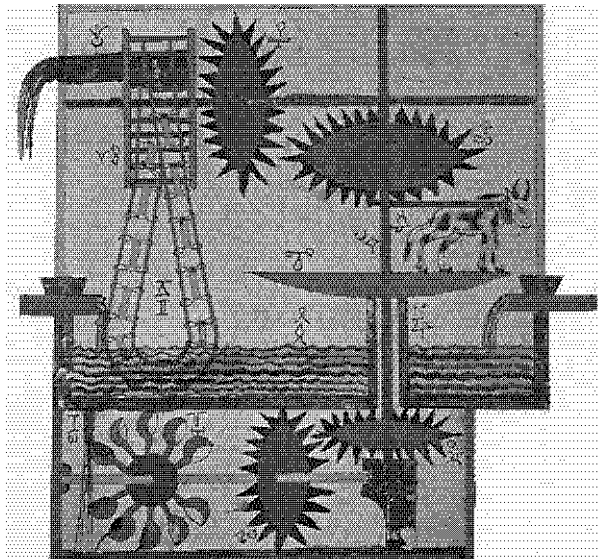
Figura 34. Representación de la sāqiya (acequia) del Tratado al-Yazari, en Ahmad Y. al Hassan, “El Islam y la ciencia”, en Mundo Científico , 17, Barcelona, Fontalba, 1982, p. 835. Lo importante de la representación no es sólo el conducto o regadera (acequia) sino “el ingenio” o “artificio” para subir o elevar el agua al que se le da el mismo nombre de regadera.
