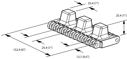
E1 Dimensions
