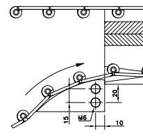
Patín de retorno
