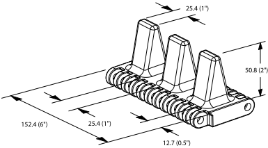
E2 Dimensions
