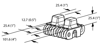
Empujadores T1
