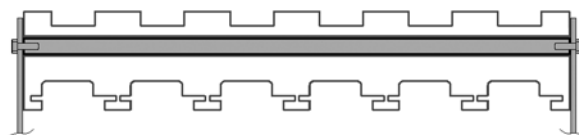
Partes Superior Y De Retorno Montadas Contra Una Barra Transversal
