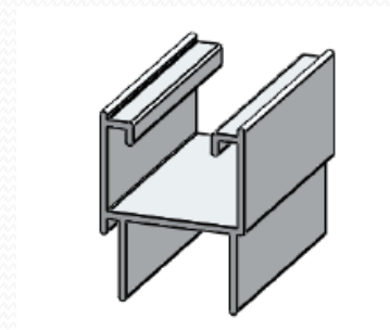
Traslape - EXA192
