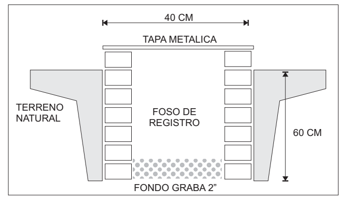
CORTE A-A
